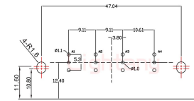
PCB布局 (PCB Layout)
